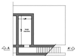
PIANTA LOCALE MACCHINE - scala 1:100
