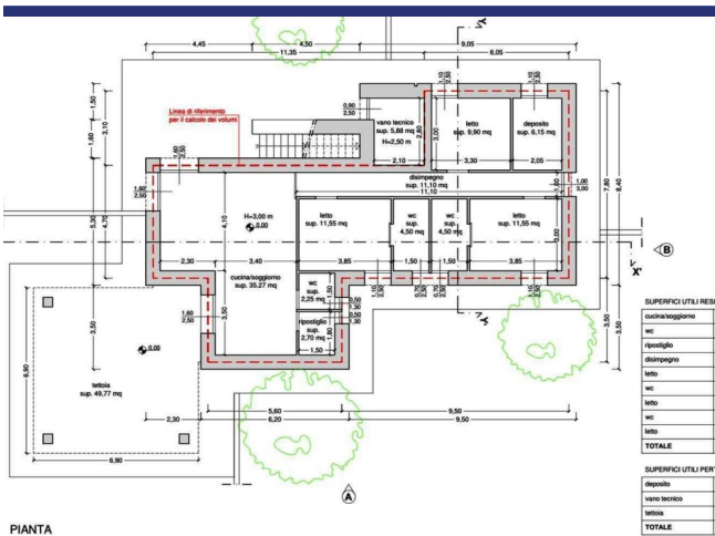
PIANTA
